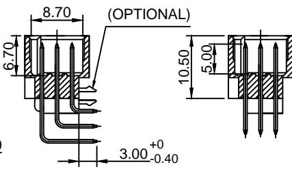
SEC A-A
